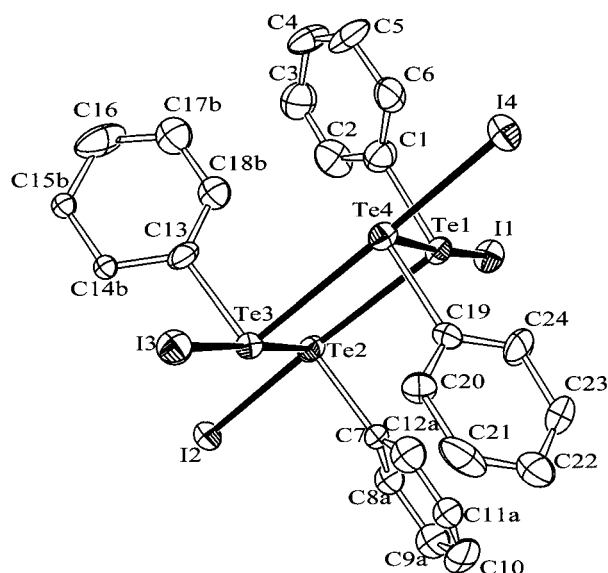
Figure 2. The X-ray crystal structure of 1 . Selected bond lengths [Å] and angles [°]: Te1–I1 2.799(2), Te2–I2 2.818(14), Te3–I3 2.822(2), Te4–I4 2.830(2), Te1–Te2 3.1474(14), Te2–Te3 3.125(2), Te3–Te4 3.1627(14), Te4–Te1 3.175(2), I1–I4 a 3.841(3), I1–I2 b 3.852(3), I2–I3 c 3.898(3), I3–I4 d 3.856(3)—where a denotes x + 1/2, y - 1/2, z ; b denotes x + 1/2, y + 1/2, z ; c denotes x + 1/2, y - 1/2, z ; and d denotes 1/2 - x, y - 1/2, z ; I1–Te1–Te(2) 94.09(4), I1–Te1–Te4 176.12(4), Te2–Te1–Te4 89.78(3), I2–Te2–Te1 175.56(5), I2–Te2–Te3 93.75(4), Te1–Te2–Te3 90.49(3), I3–Te3–Te2 175.77(4), I3–Te3–Te4 93.70(4), Te2–Te3–Te4 90.40(3), I4–Te4–Te1 93.92(4), I4–Te4–Te3 176.77(5), Te1–Te4–Te3 89.31(3).
